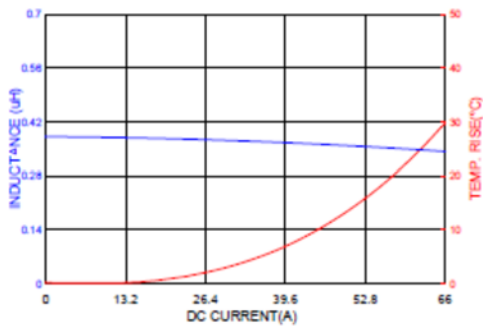
HMPL1265HP-R36
